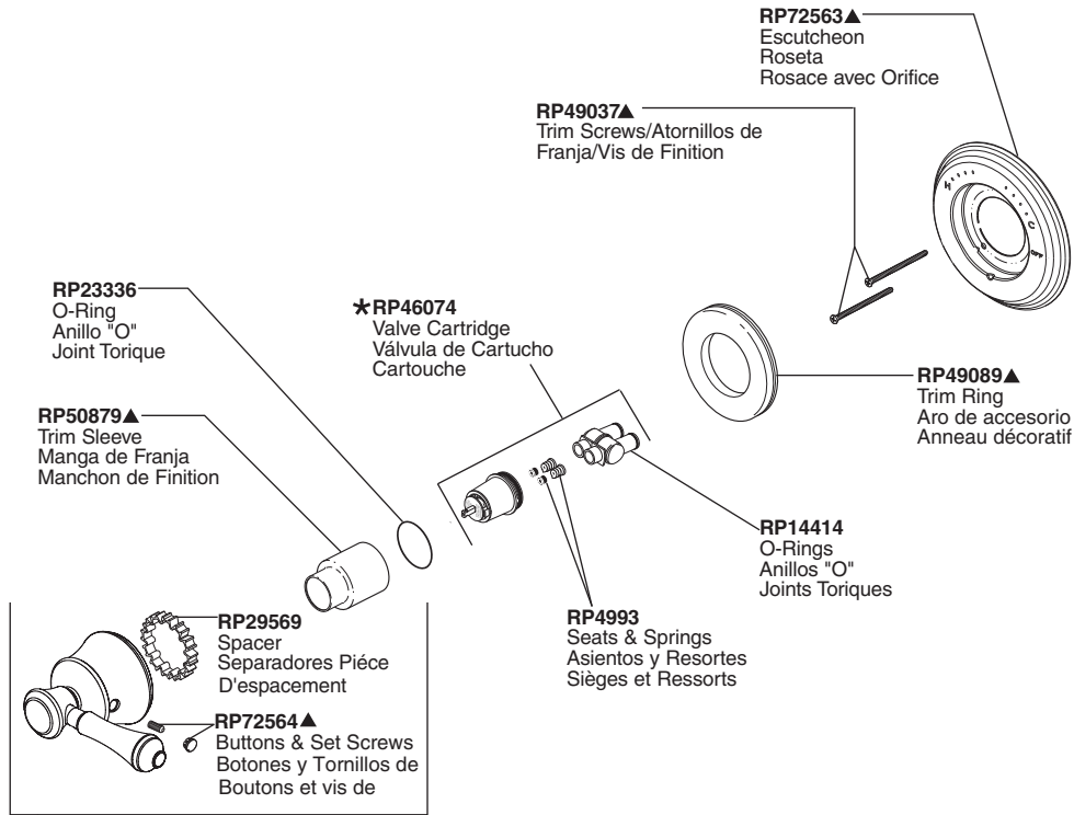
H797▲ Handle Kit Juego de herrajes de la Manija Manette en kit
