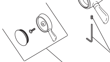
RP51309▲ Temperature Knob, Cover & Screw Perilla de la Temperatura, Cubierta y Tornillo Poignée de Réglage de Température et Vis
