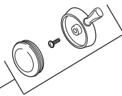
RP61276▲ Temperature Knob, Cover & Screw Perilla de la Temperatura, Cubierta y Tornillo Poignée de Réglage de Température et Vis
