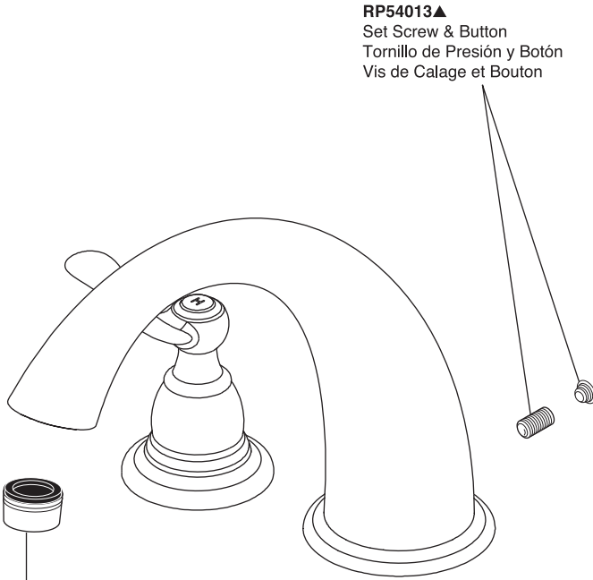
RP47419▲ Stream Straightener Kit Enderezador del chorro Concentrateur de jet
