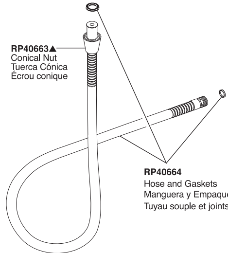
RP46683▲ Hand Piece Pieza de Mano Douche à main
